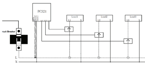
Schéma zapojení jednofázové elektřiny
