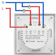
SCHÉMA ZAPOJENÍ
